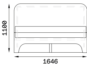
Con testata (a filo)
